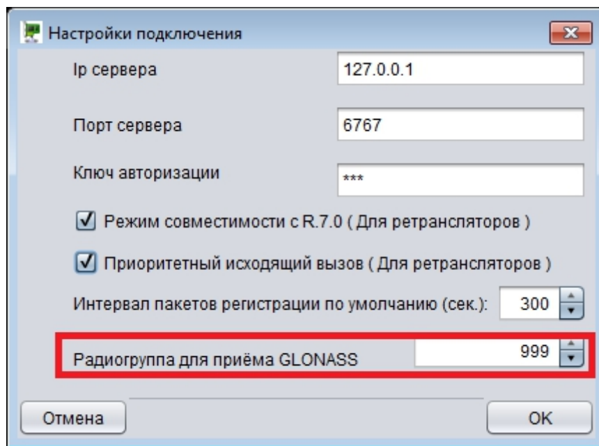
Рисунок 17.8 – ПО «Шлюз DMR». Настройка «Радиогруппы» для приема ГЛОНАСС/GPS координат
