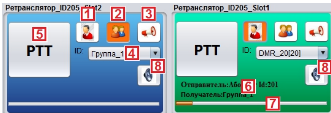
Рисунок 12.5 – Панель управления приемопередатчиком (трансивером)
