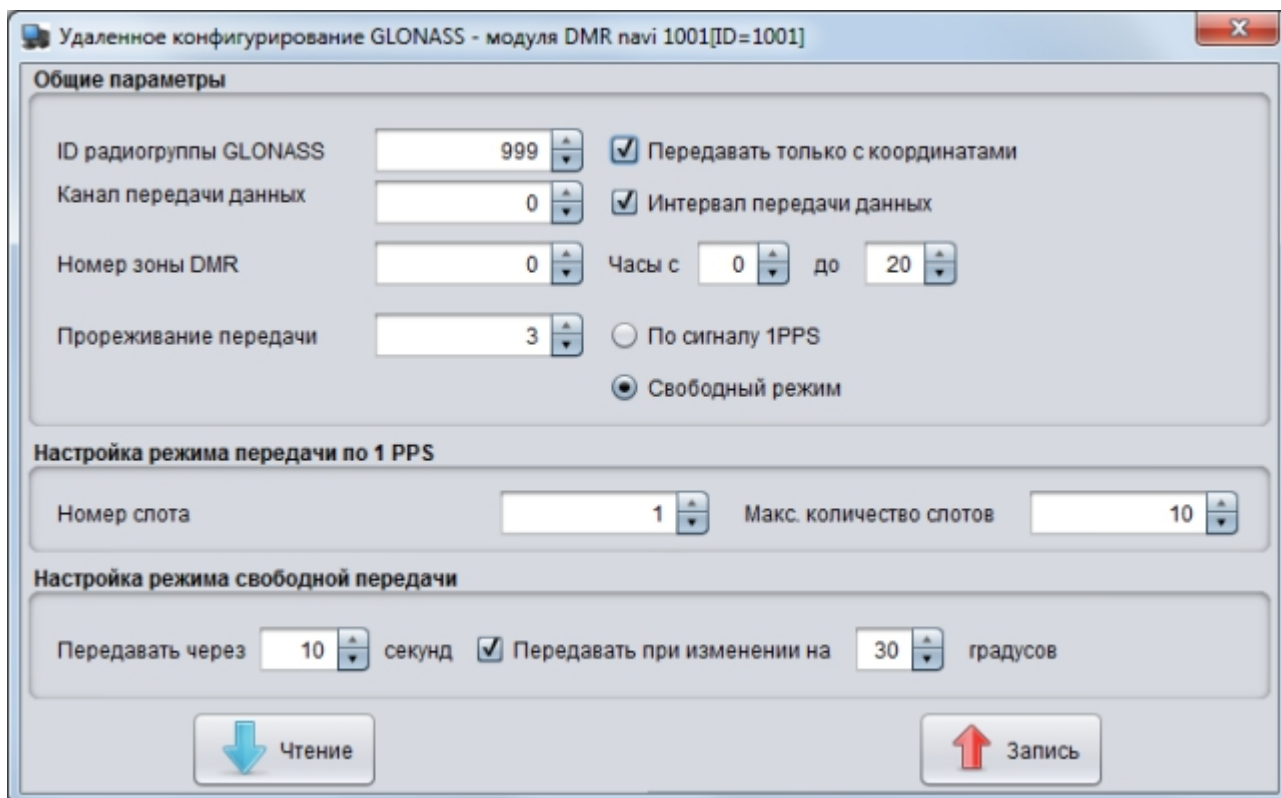
Рисунок 17.7 – Панель настройки ГЛОНАСС/GPS
