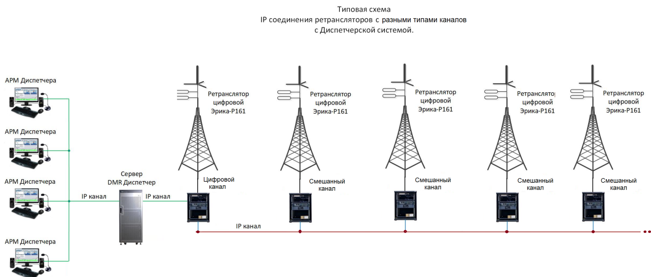
Рисунок М.1 – Схема IP соединения ретрансляторов с разными типами каналов
